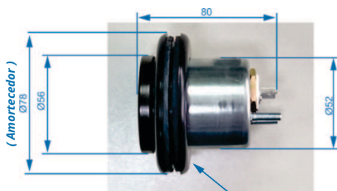
Amortecedor (DNI 4502)
